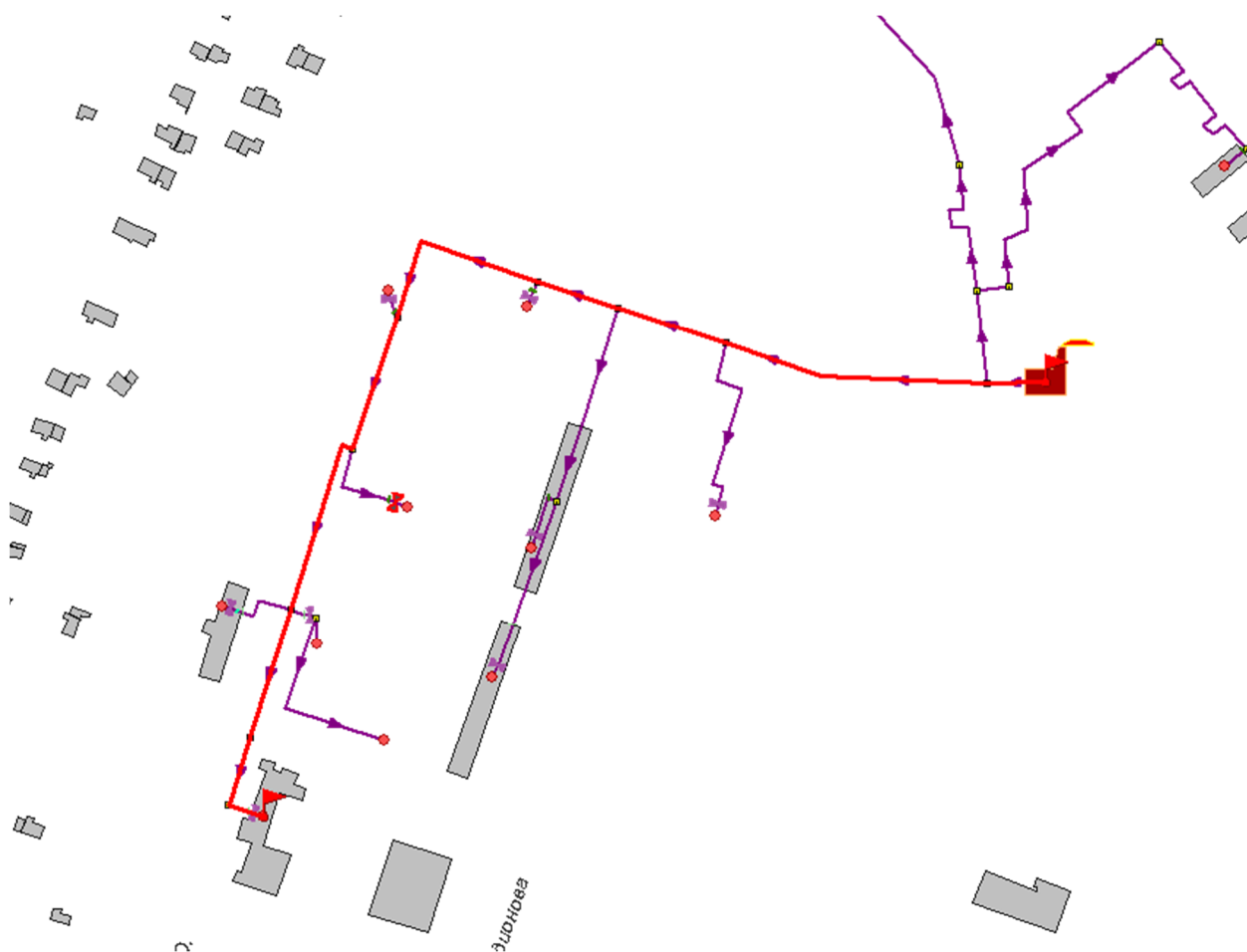
Рисунок 2.87 -Расчетный путь теплоносителя от котельной до Капитана Храмцова,5а
