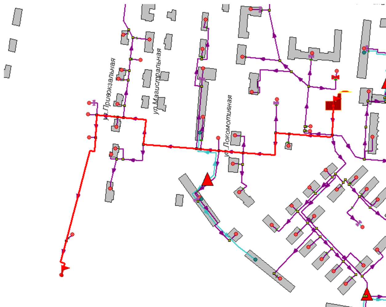
Рисунок 2.43 -Расчетный путь теплоносителя от котельной до Привокзальная, 19
