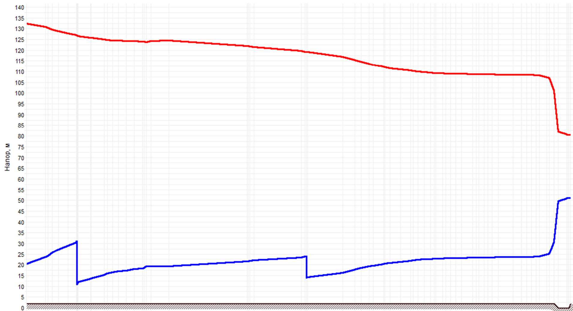
Рисунок 2.4 –График гидравлических режимов рассматриваемого теплопровода
