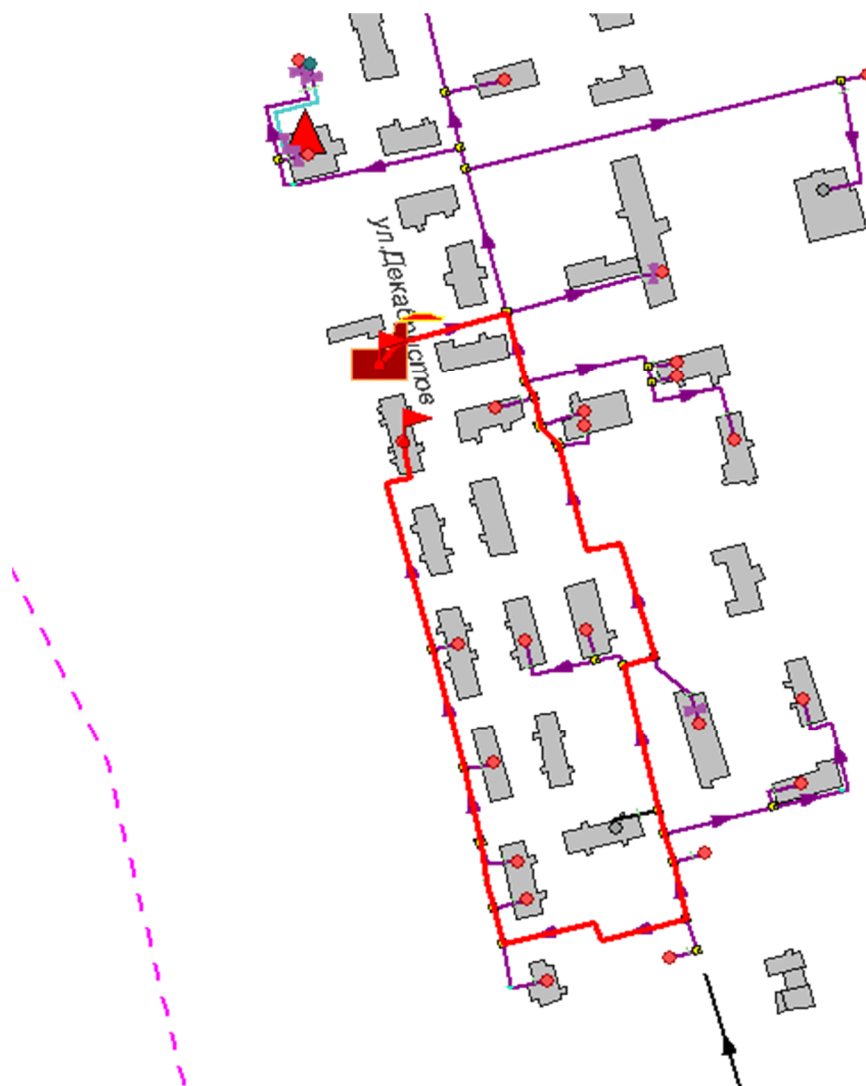
Рисунок 1.57 -Расчетный путь теплоносителя от котельной до Декабристов, д. 15
