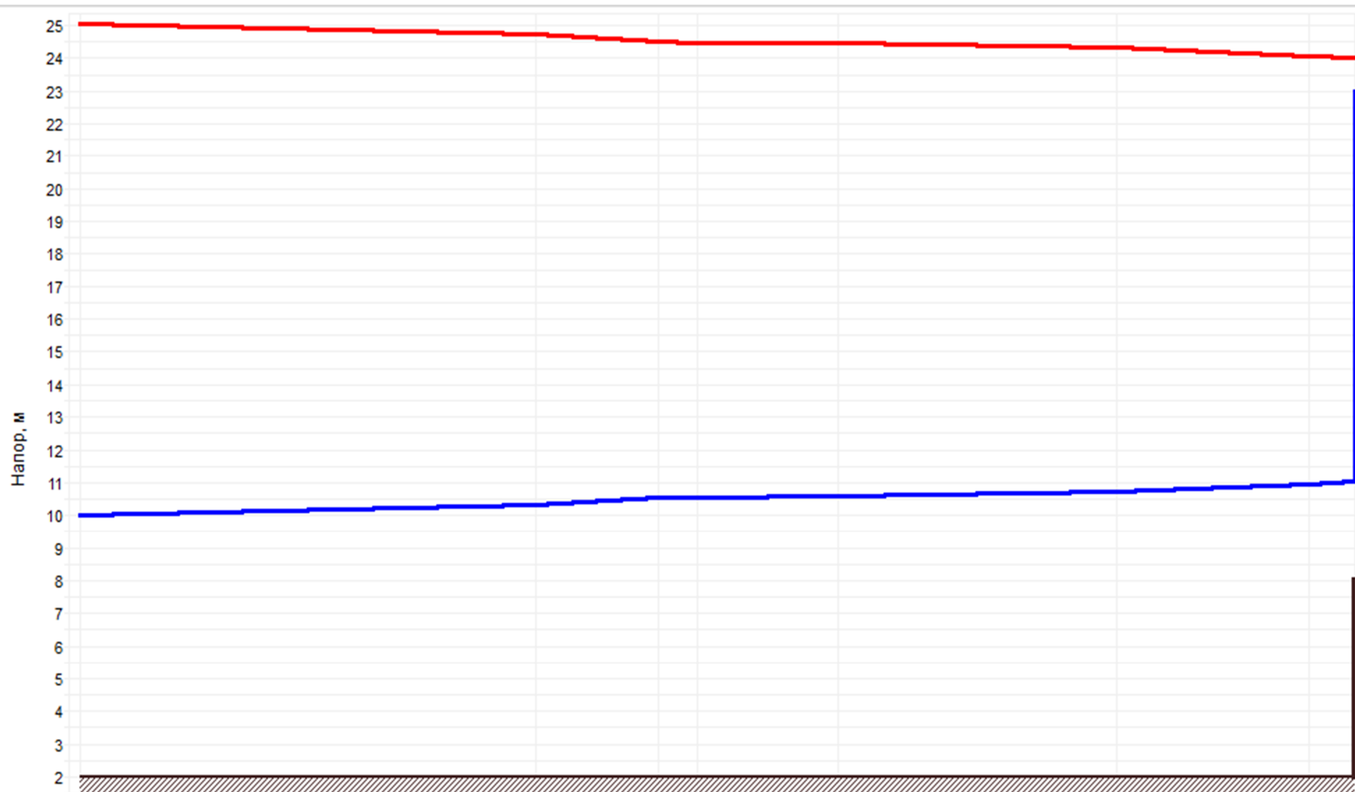
Рисунок 3.74 –График гидравлических режимов рассматриваемого тепловпровода
