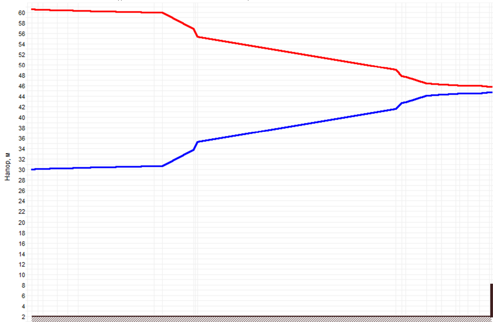
Рисунок 1.20 –График гидравлических режимов рассматриваемого теплопровода
