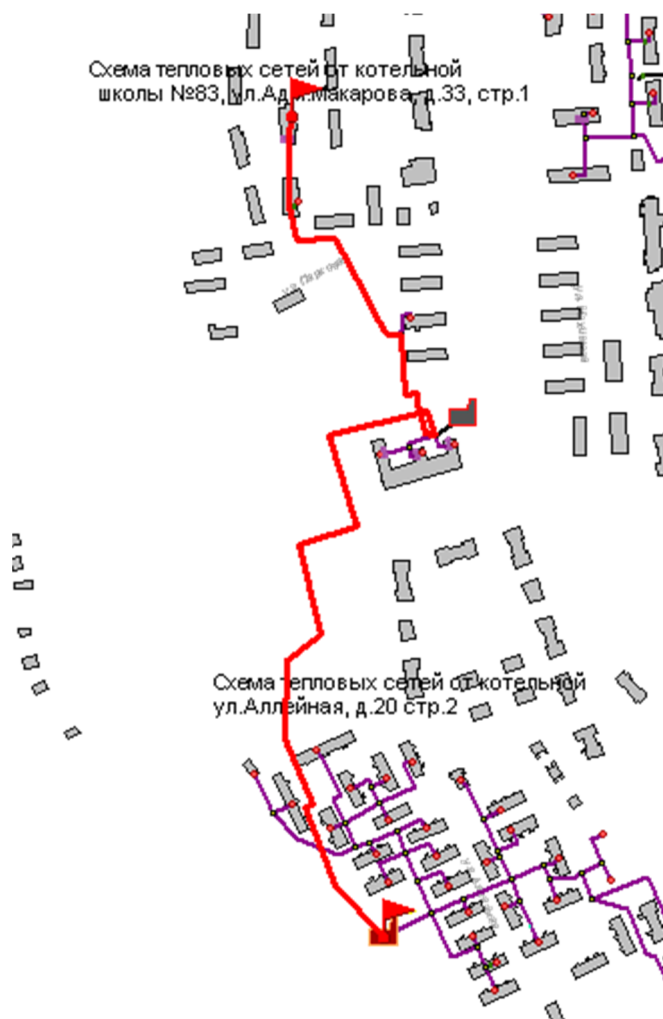
Рисунок 1.27 -Расчетный путь теплоносителя котельной до КИЗ «ЛУЧ»
