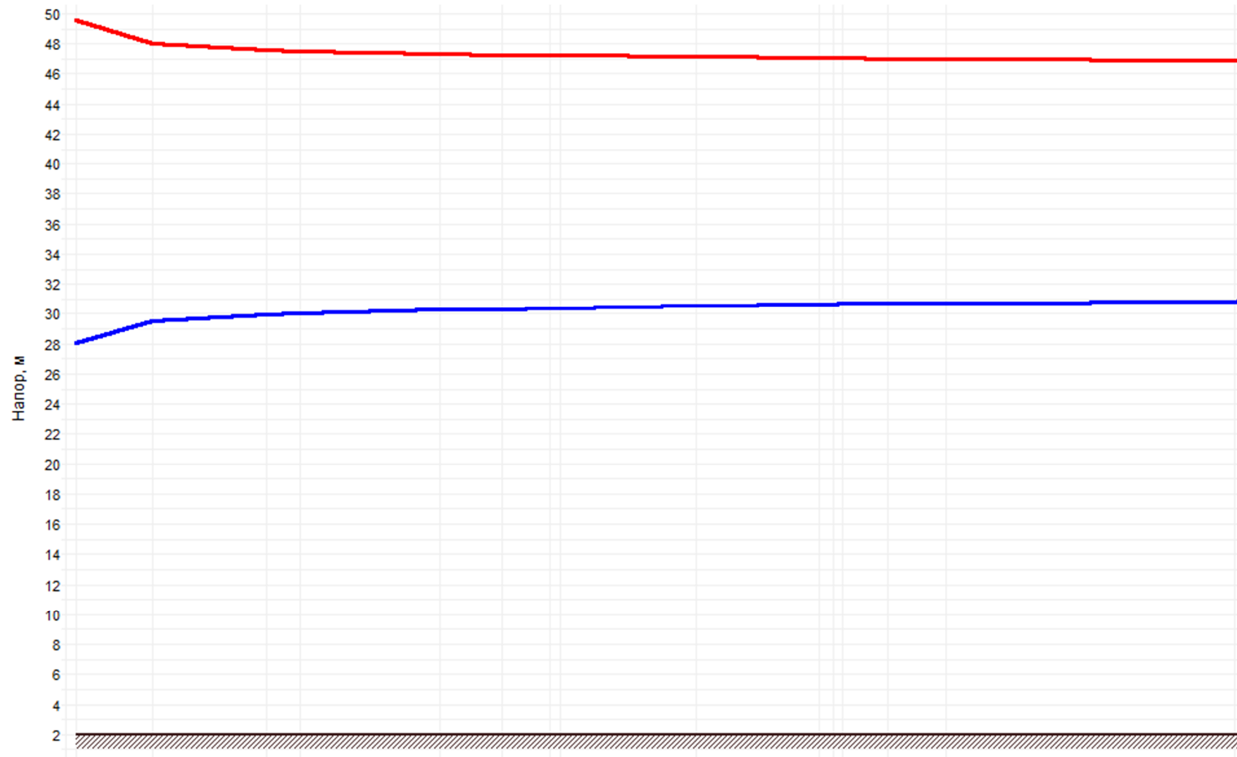
Рисунок 3.44 –График гидравлических режимов рассматриваемого теплопровода
