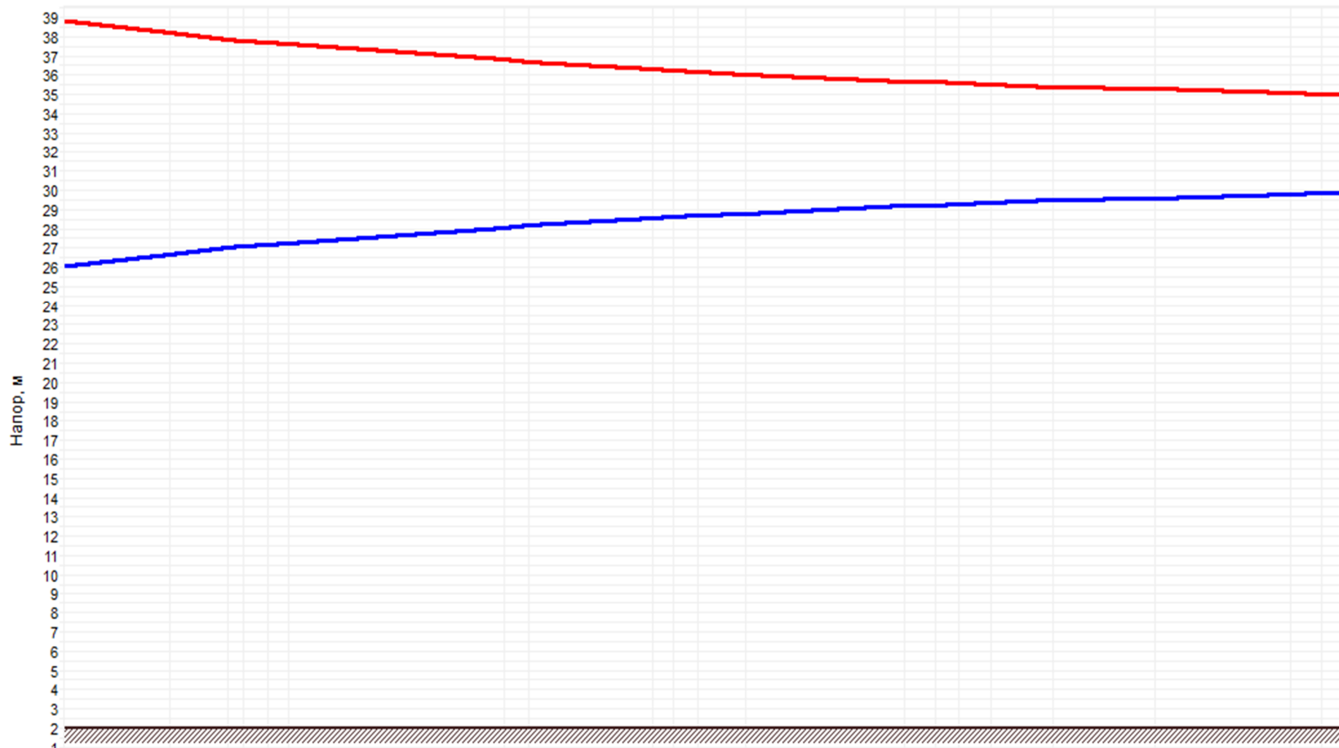
Рисунок 1.58 –График гидравлических режимов рассматриваемого теплопровода
