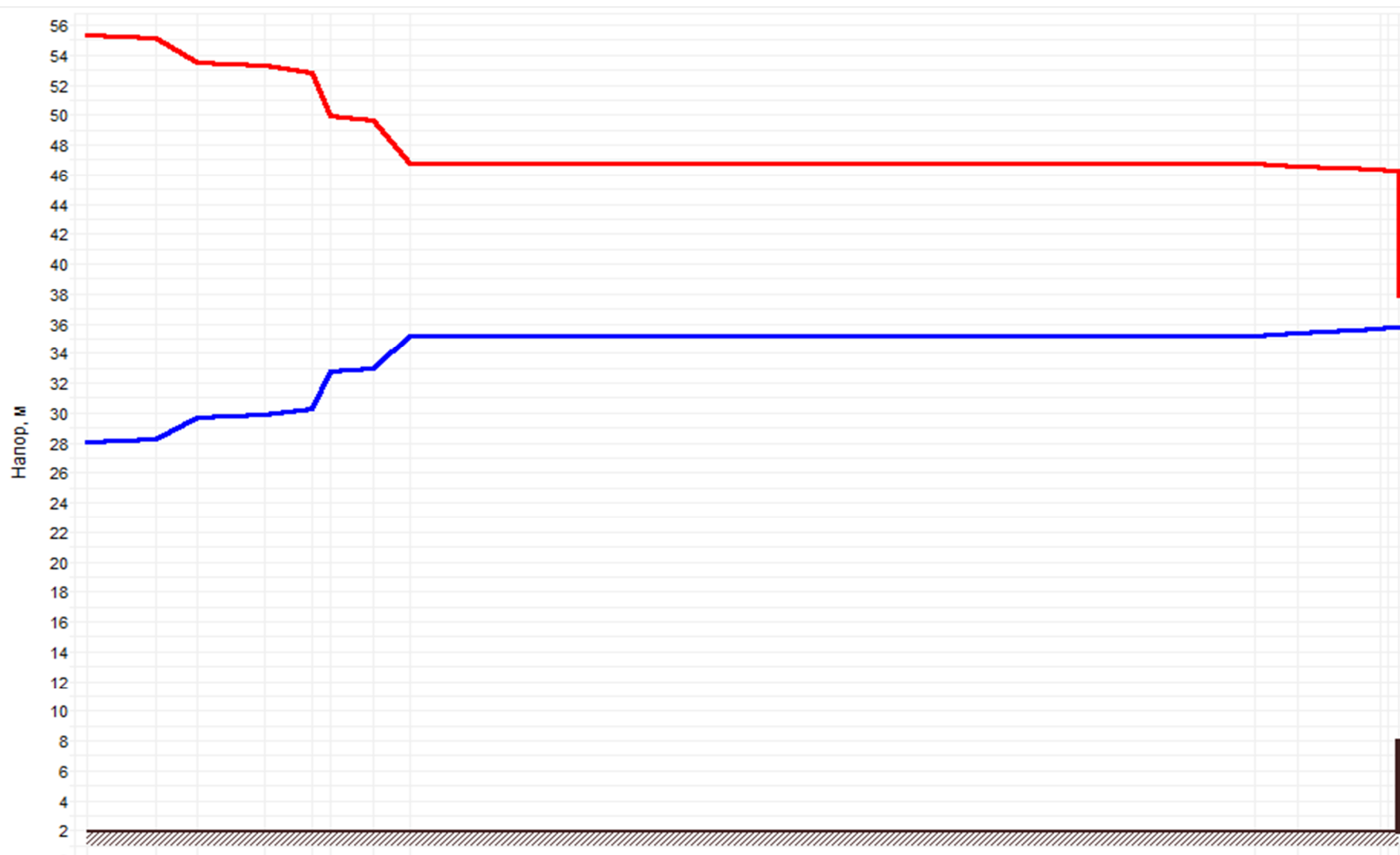
Рисунок 3.30 –График гидравлических режимов рассматриваемого теплопровода
