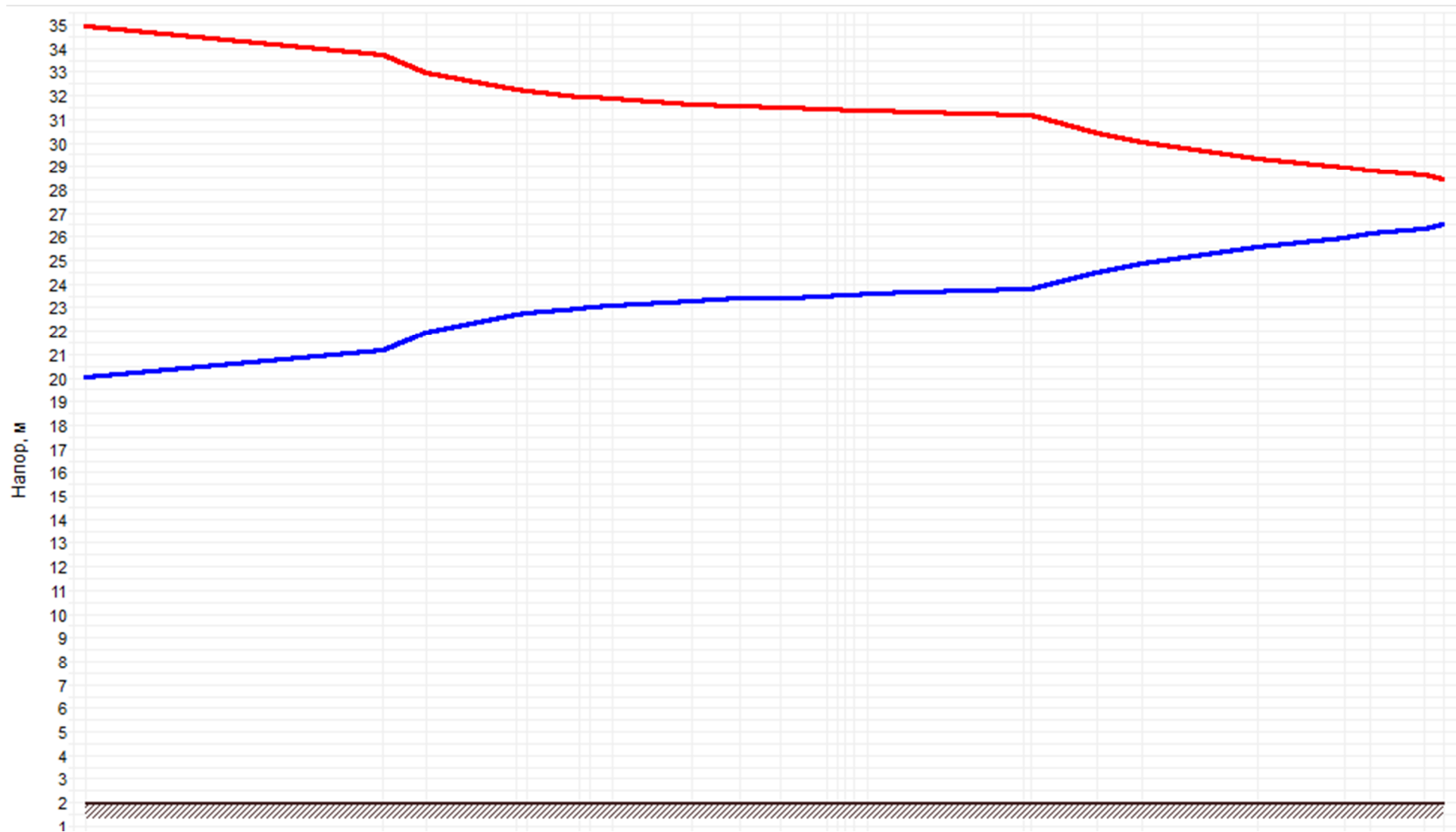
Рисунок 1.66 –График гидравлических режимов рассматриваемого теплопровода
