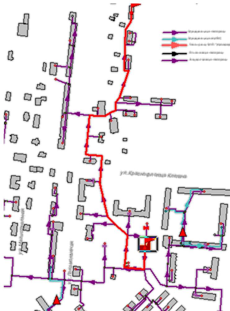
Рисунок 3.45 -Расчетный путь теплоносителя от котельной до Локомотивная,1
