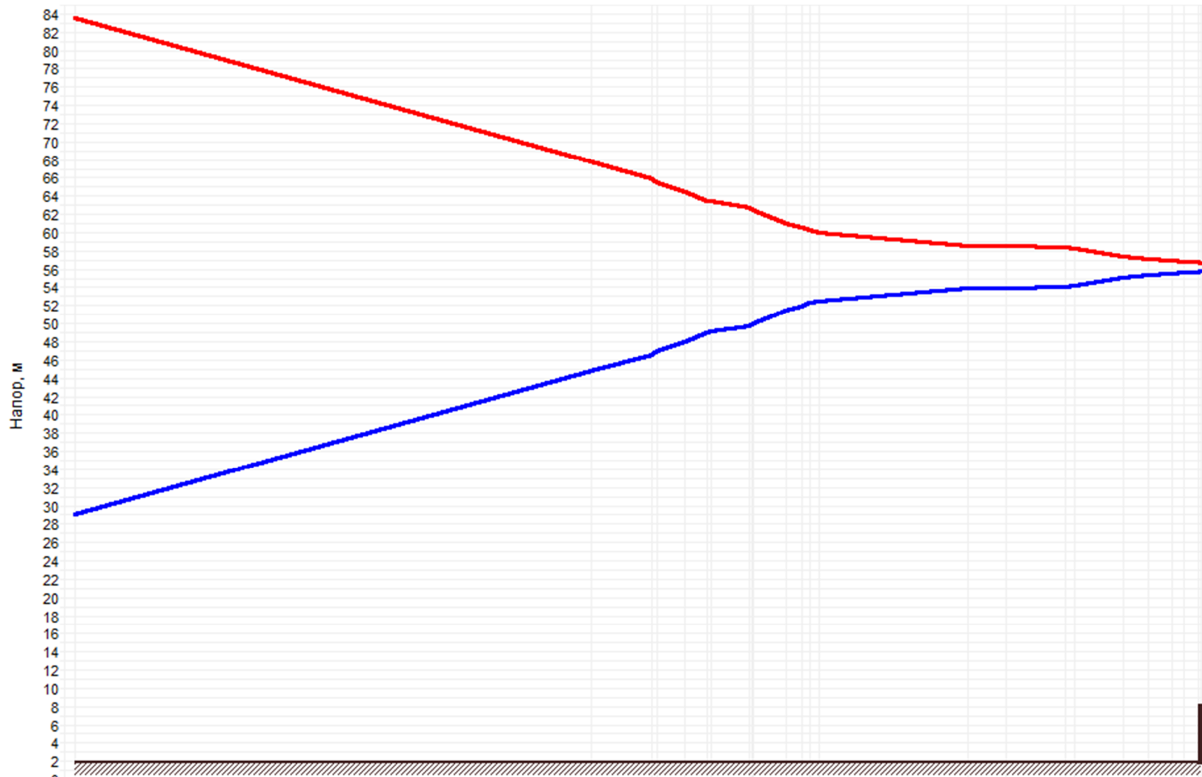
Рисунок 2.24 –График гидравлических режимов рассматриваемого теплопровода
