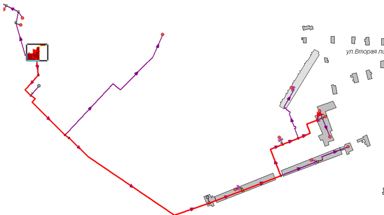
Рисунок 3.41 -Расчетный путь теплоносителя котельной до 2-я линия,9
