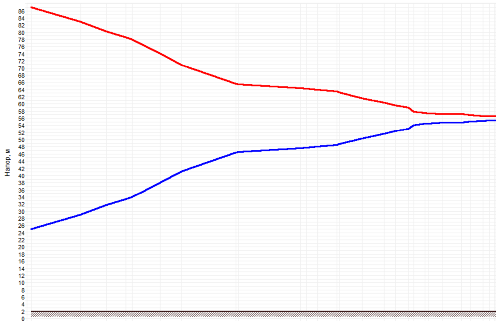
Рисунок 3.36 –График гидравлических режимов рассматриваемого тепловпровода
