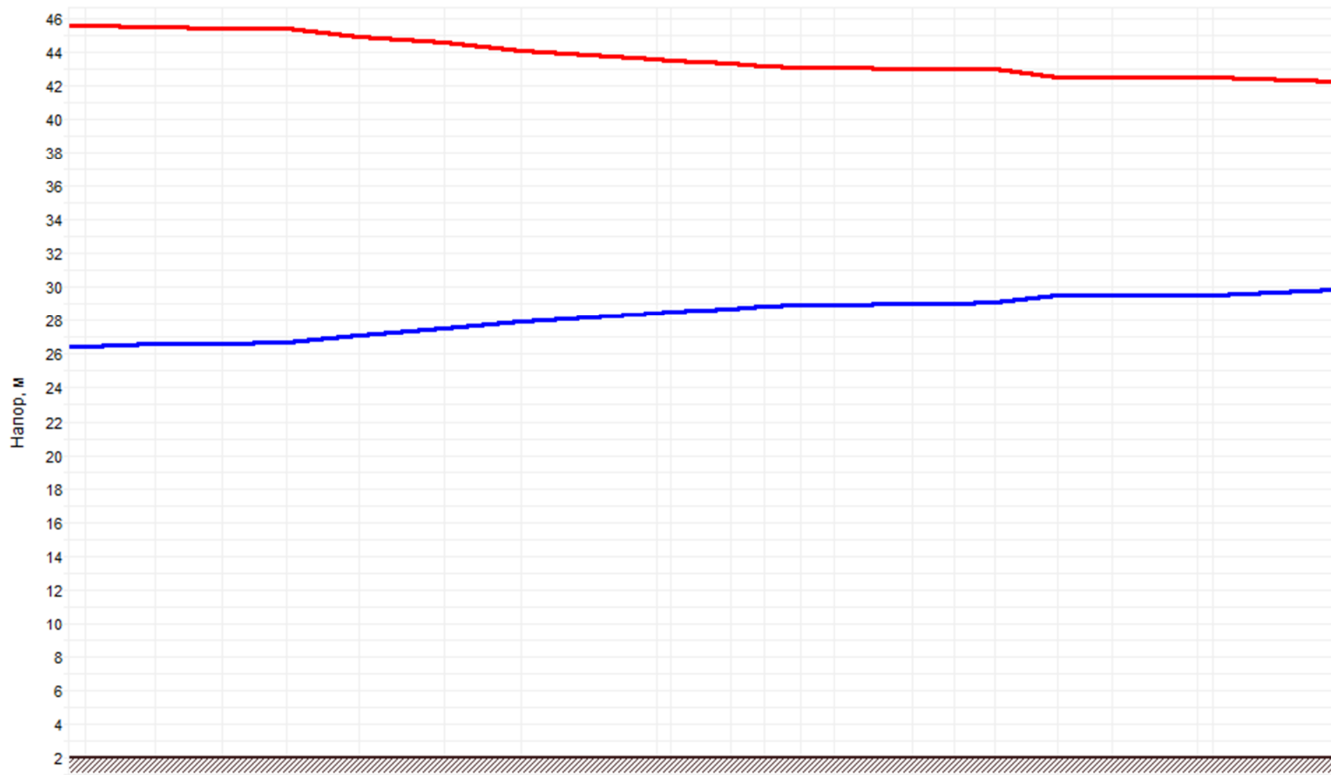
Рисунок 3.16 –График гидравлических режимов рассматриваемого теплопровода
