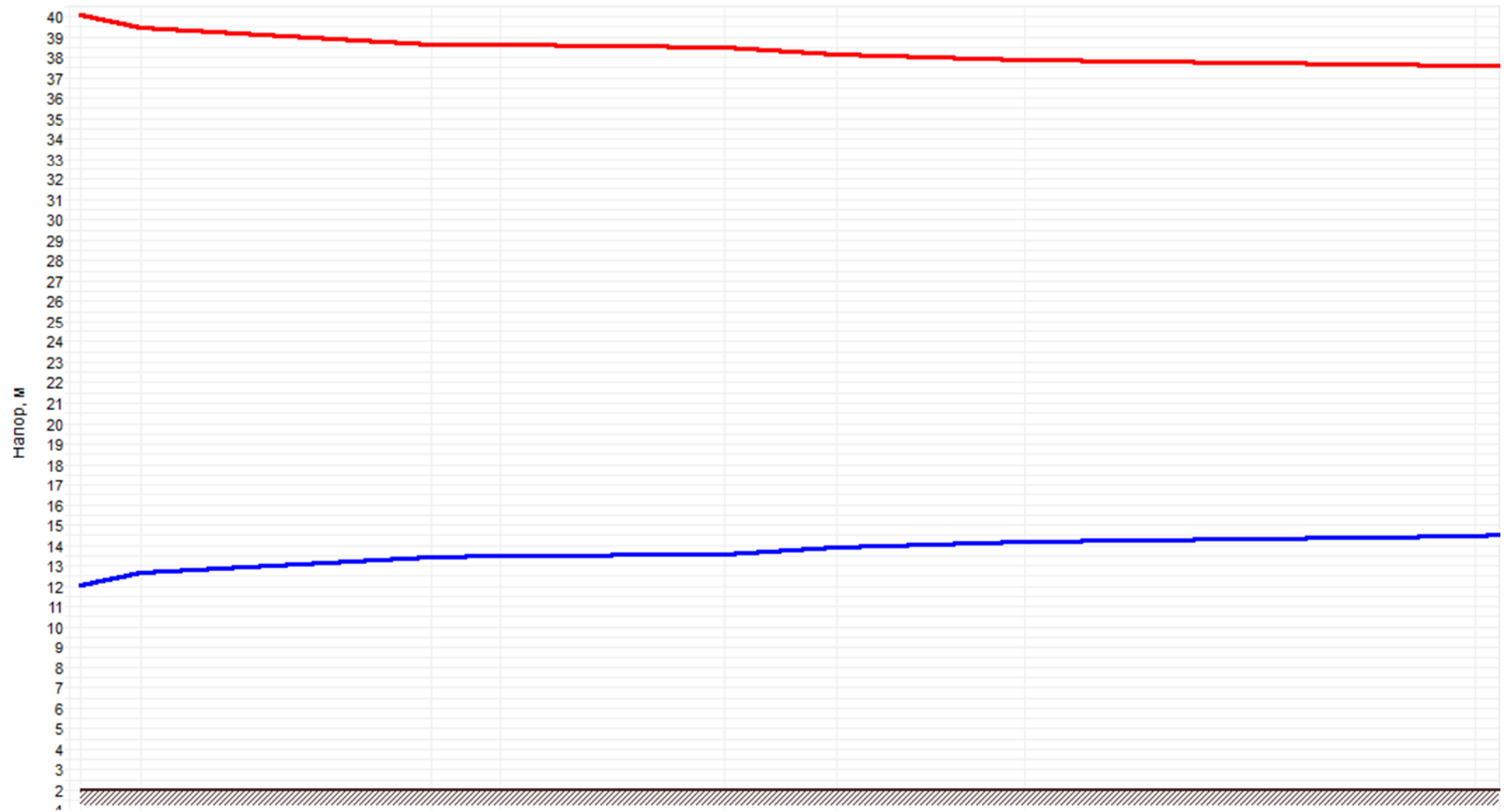
Рисунок 3.48 –График гидравлических режимов рассматриваемого теплопровода
