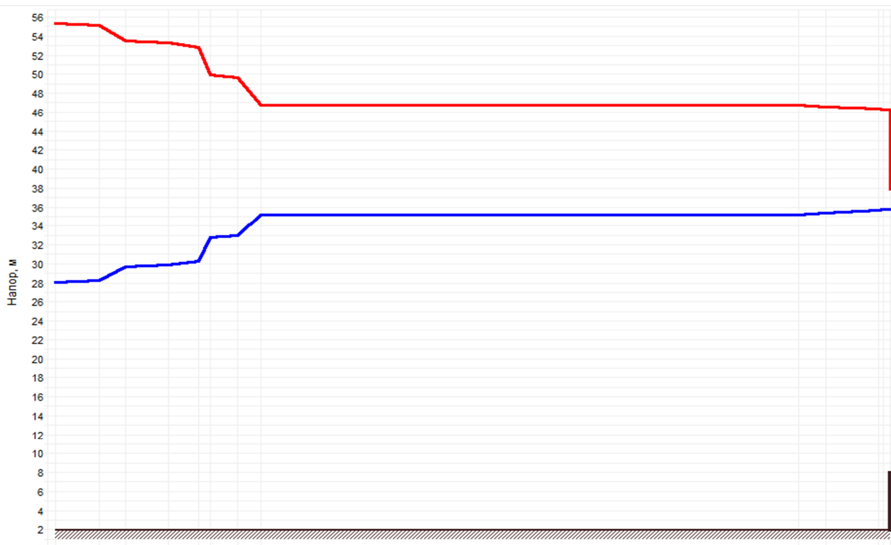
Рисунок 2.30 –График гидравлических режимов рассматриваемого теплопровода
