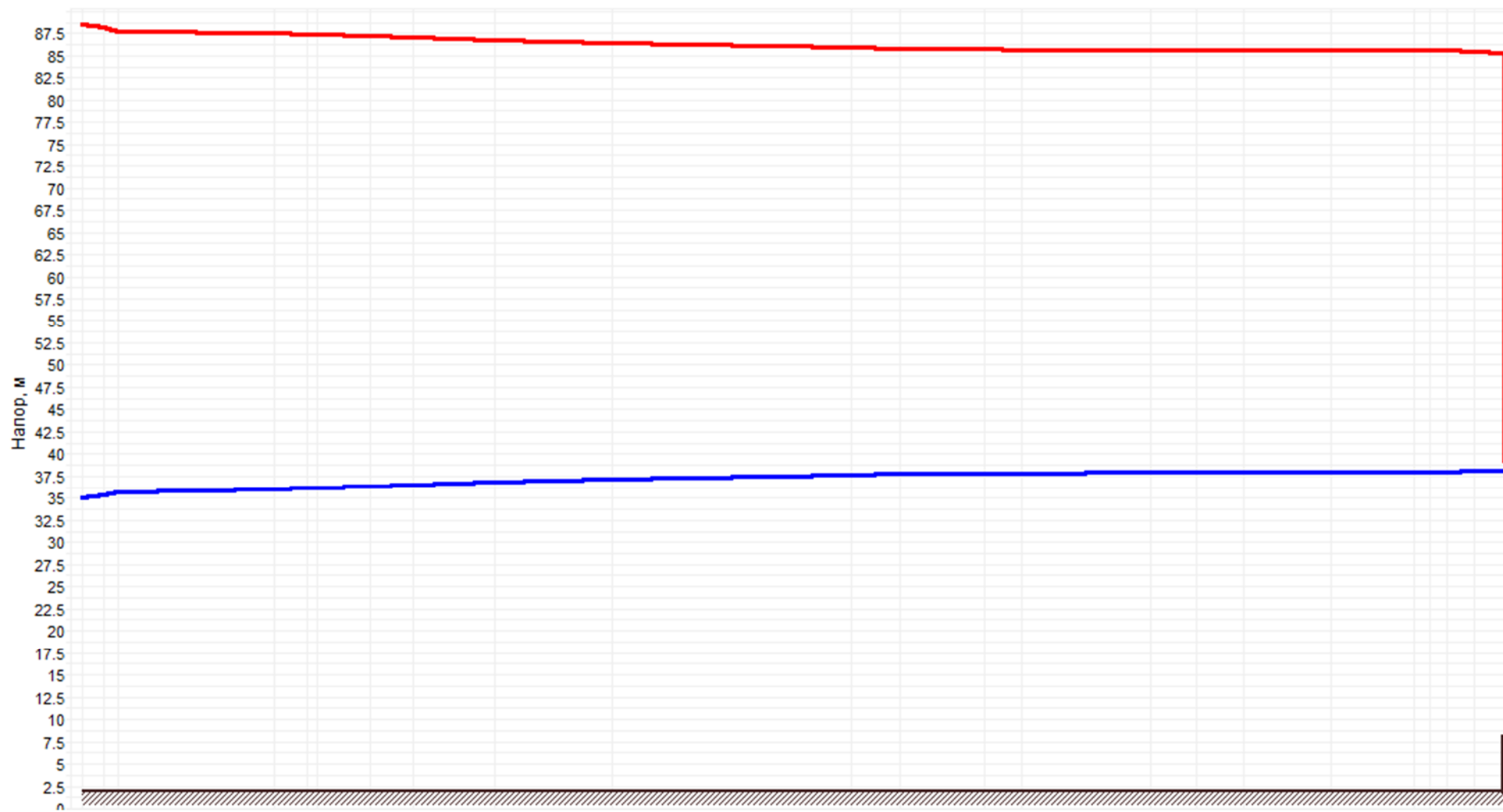
Рисунок 1.84 –График гидравлических режимов рассматриваемого теплопровода
