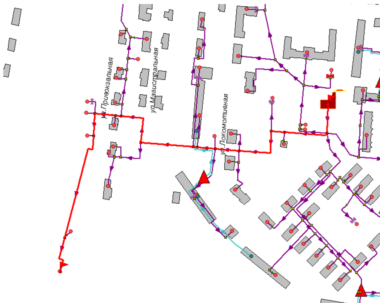
Рисунок 3.43 -Расчетный путь теплоносителя от котельной до Привокзальная, 19
