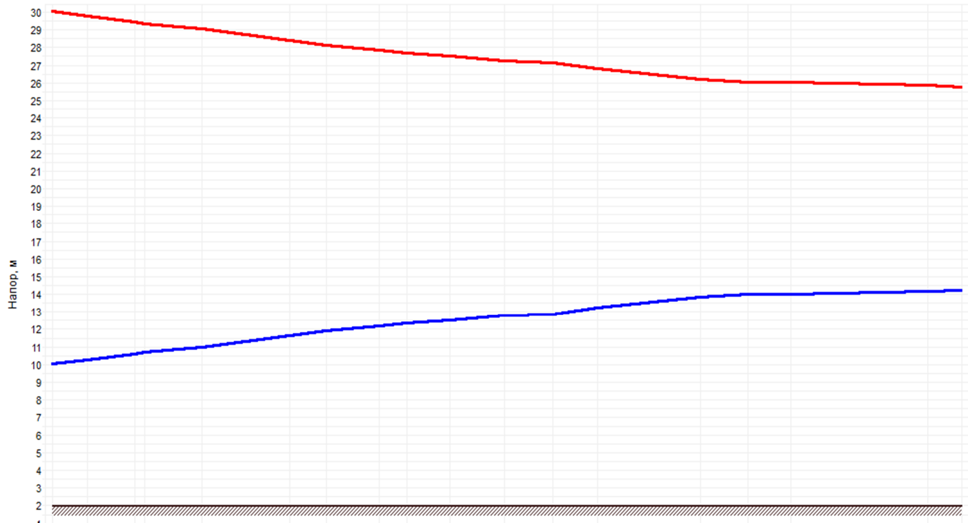
Рисунок 2.72 –График гидравлических режимов рассматриваемого теплопровода
